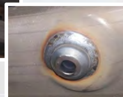
MIG WELDS
